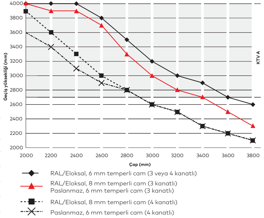
KTV 3/4 standart kanat için çap/yükseklik tablosu
