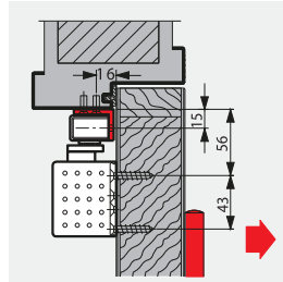
Binili kapılarda kasa kayar kolu montajına elverişli değilse 90° montaj plakası kullanılabilir.
