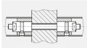
MIM-432-00-052 GZ 214 (28-75 mm) Ahşap/metal kapılar için çift taraflı bağlantı elemanı
