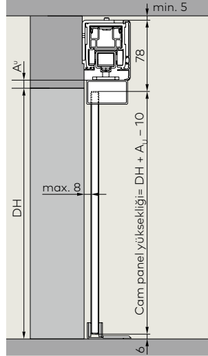
Cam kanat / cam sıkıştırma rayı (duvar üzerinde)
