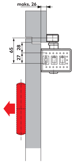
İtme yönünde kanada montaj
