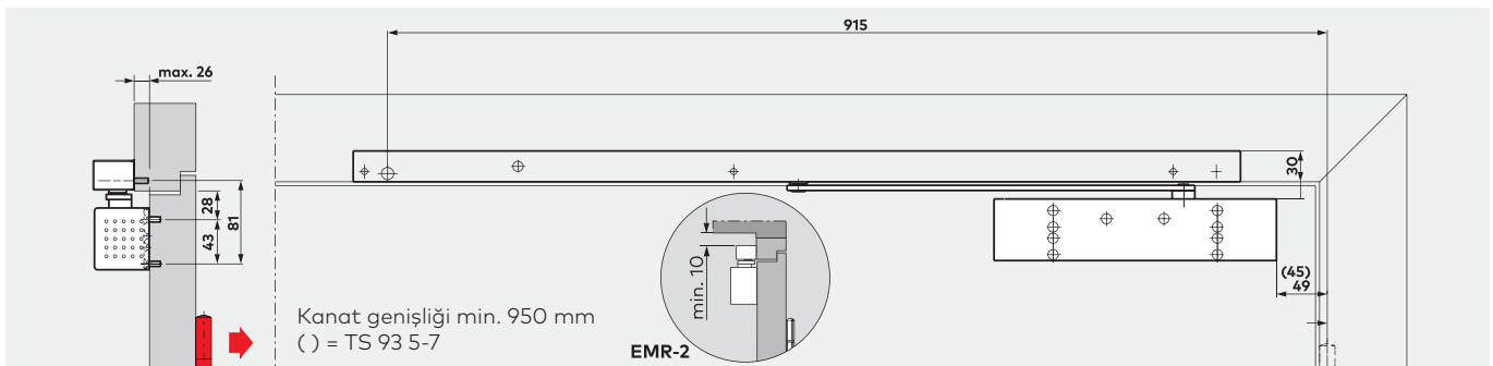
TS 93 B - EMR, kapı kanadına itme yönünde montaj
