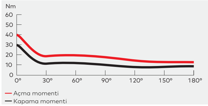
Kapı kanadına çekme yönünde montaj TS 92 B Yaklaşık 180° açılma olanağı sağlar.
