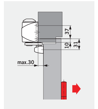
Kapı kasasına itme yönünde montaj
