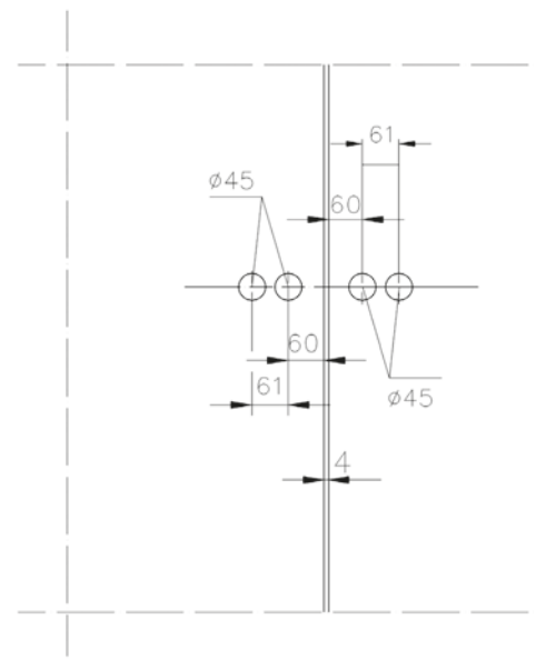
Studio Rondo cam cama kilit karşılık cam delik detayı
