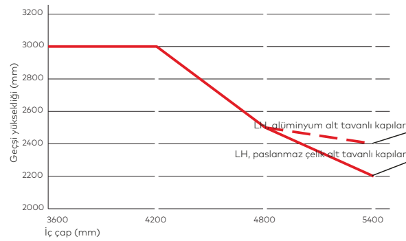
KTC 2 Çap/yükseklik tablosu
