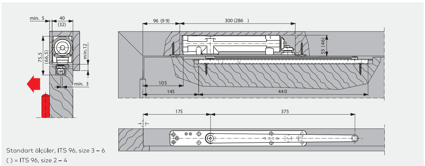
ITS 96 ahşap kapı uygulaması
