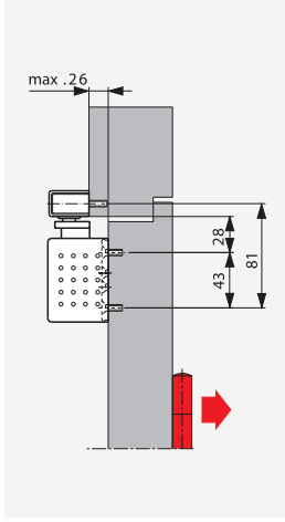
Kapı kanadına çekme yönünde montaj TS 92 G Yaklaşık 180° açılma olanağı sağlar.
