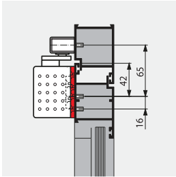
Montaj plakası uygulaması kapatıcının direk montajı mümkün değilse.
