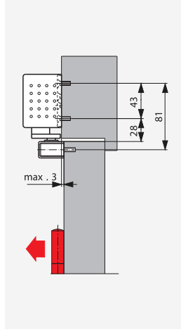
Kapı kanadına itme yönünde montaj TS 92 G Yaklaşık 120°-145° açılma olanağı sağlar.
