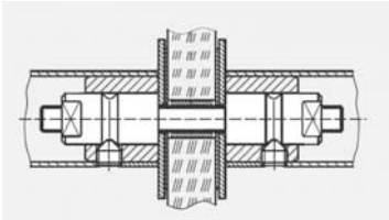
MIM-432-00-047 GZ 215 (8-15 mm) Cam kapılar için çift taraflı bağlantı elemanı
