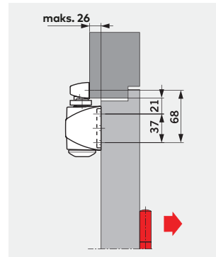
Kapı kanadına itme yönünde montaj
