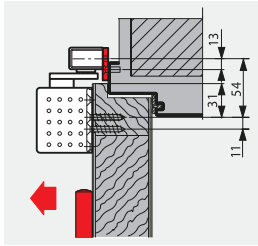
Kayar kol için ekstra montaj plakası
