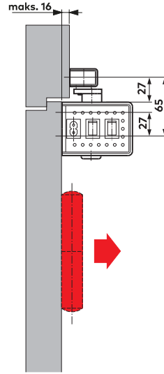
Çekme yönünde kanada montaj
