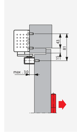
Kapı kanadına itme yönünde montaj TS 92 B Yaklaşık 120°-145° açılma olanağı sağlar.
