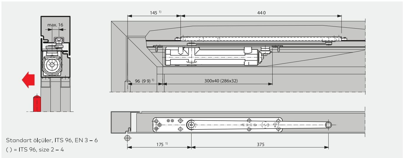
ITS 96 alüminyum kapı uygulaması
