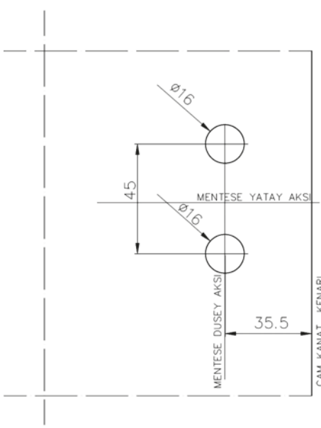
Arcos Office menteşe cam delik detayı
