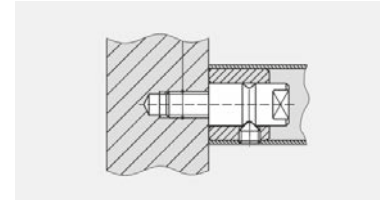
MIM-432-00-121 GZ 234 Çerçevesi kapılar için (20mm vida derinliği) Tek taraflı bağlantı elemanı
