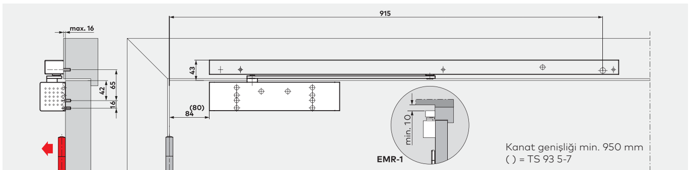
TS 93 B - EMR, kapı kanadına çekme yönünde montaj
