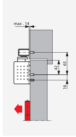
Kapı kanadına çekme yönünde montaj TS 92 B Yaklaşık 180° açılma olanağı sağlar.
