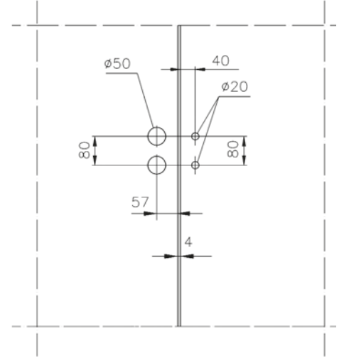
Arcos Office cam cama kilit karşılığı cam delik detayı
