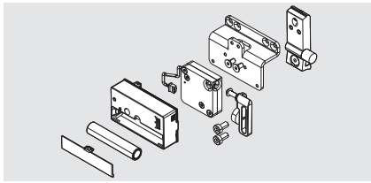
MIC-422-00-270 Elektromekanik kilit
