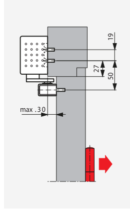
Kapı kanadına itme yönünde montaj Yaklaşık 120°-145° açılma olanağı sağlar.
