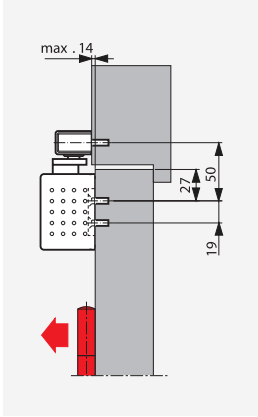
Kapı kanadına çekme yönünde montaj Yaklaşık 180° açılma olanağı sağlar.
